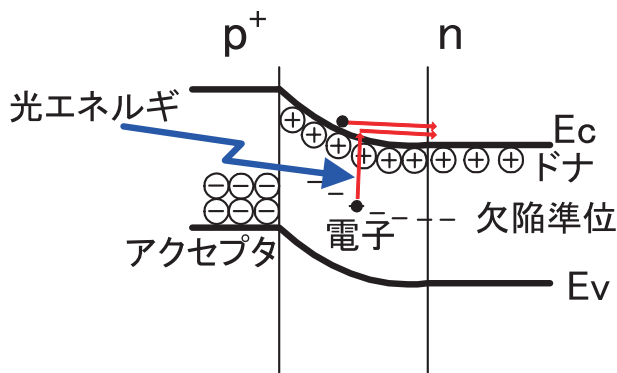
フォトキャパシタンス測定原理
